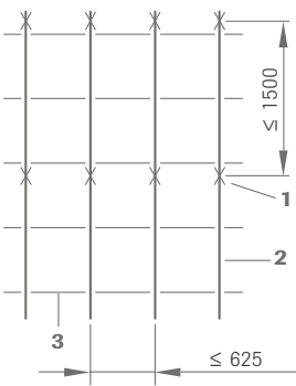
Module 625 x 625 mm
