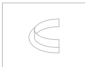
Nr. 8034/1' Säulenanschluss Halbring Ø 250 – 500 mm in 50er Schritten; Höhe: 20 mm, Breite: 20 mm; Dicke: 1,5 mm
