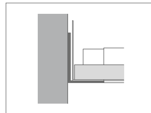
Nr. 51/1 Bandraasterdecken System S 18p/k
