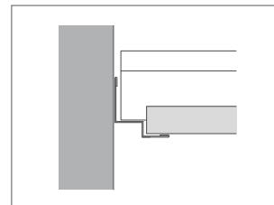
Nr. 50/15 Contura-Decken, System S 3a und System S 15a cliq
