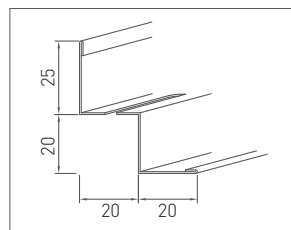
Nr. 56/35 0,6 mm dick (mit Lüftungsschlitzen)
