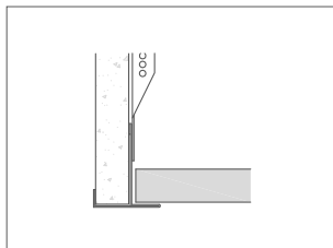
Nr. 8030/13, Nr. 8030/15 Deckenversprung oder Abschottung
