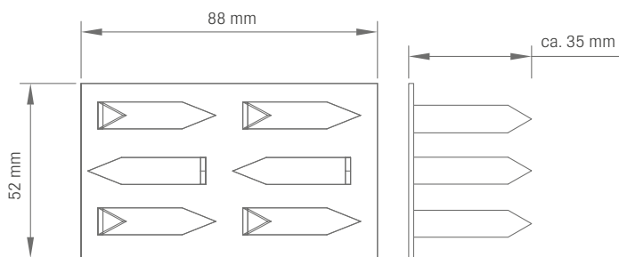
6 Wandkralle für 40 mm starken Wandabsorber, Krallenhöhe 35 mm
