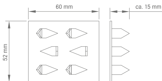
6 Wandkralle für 40/20 mm starken Wandabsorber, Krallenhöhe 15 mm
