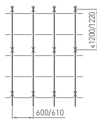
Module 3 600 x 600 mm 610 x 610 mm (2'x 2')
