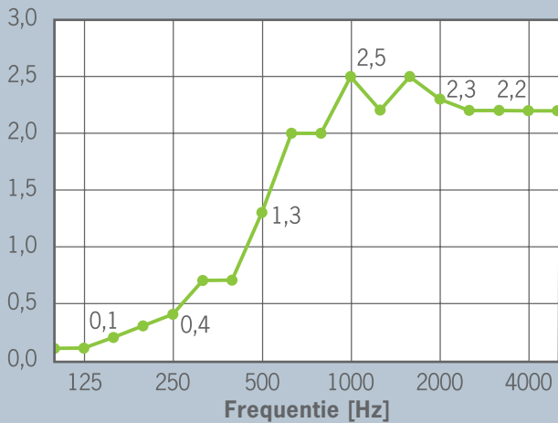
Equivalent geluidsabsorptieoppervlak [m 2 ] OWAcoustic® vela (H = 415 mm)
