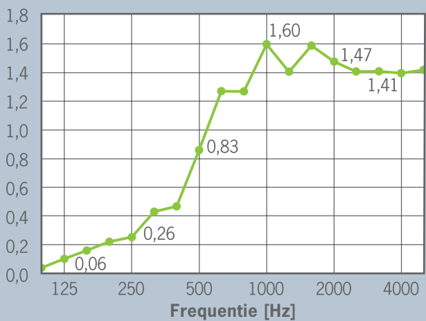
Geluidsabsorptiegraad \alpha_s OWAcoustic® vela (H = 415 mm)
