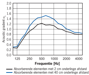
HDF/MDF-paneel met vierkante perforatie QP 10/22,5 met een vrije doorlaat van 20,7 %
