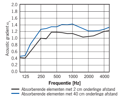
OWAcoustic®-plaat met vliesbekleding en Creaprintbedrukking
