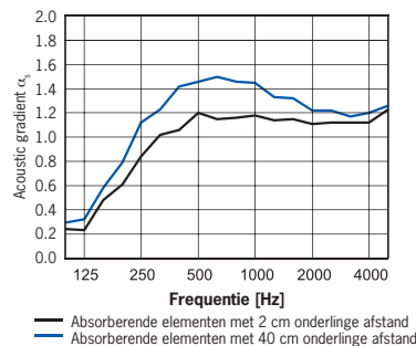
Aluminium met vierkante perforatie QL 5/8 met een vrije doorlaat van 39,1 %
