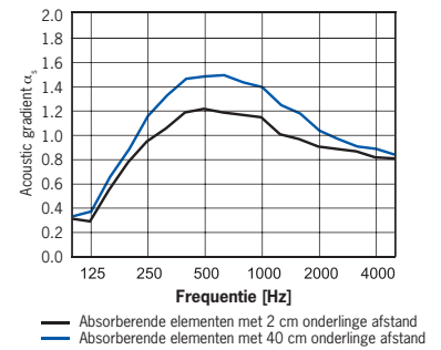
Aluminium met ronde perforatie RL 2.5/8.0 met een vrije doorlaat van 7,6 %
