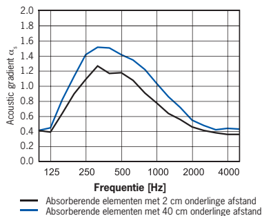
OWAtecta® perfora met een vrije doorlaat van 0,64%
