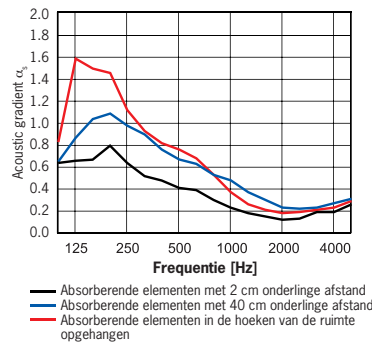
Ongeperforeerd aluminium d = 1,5 mm
